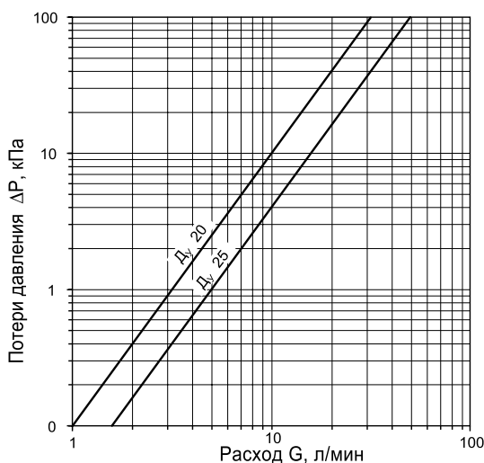
Гидравлические потери в клапане TVM-N
