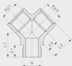
Двойной соединительный элемент - латунь Модель 1641
