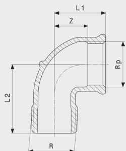
Отвод 90° - бронза Модель 3092
