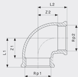
Отвод 90° - бронза Модель 3090
