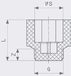
Контрольная заглушка - пластик Модель 1516.512
