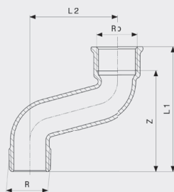
Отступ - бронза Модель 3004
