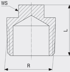
Заглушка - бронза Модель 3291
