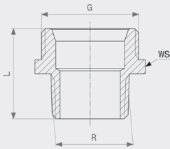
Ниппель-переход - бронза Модель 3246
