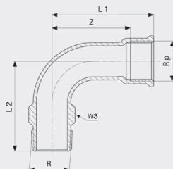
Отвод 90° - бронза Модель 3001
