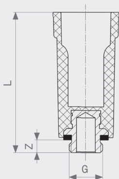
Контрольная заглушка - пластик Модель 1516.113
