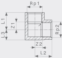
Водорозетка - латунь Модель 1421
