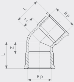
Отвод 45° - латунь Модель 1614
