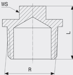
Заглушка - бронза Модель 3290
