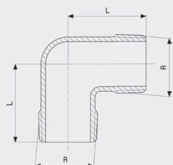
Угольник 90° - бронза Модель 3091
