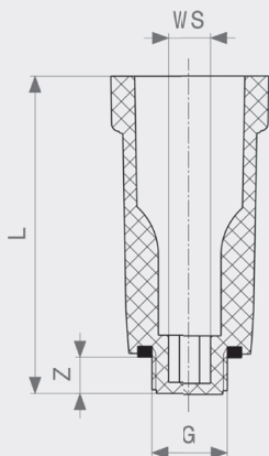
Контрольная заглушка - пластик Модель 1516
