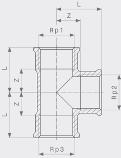
Тройник - латунь Модель 1622
