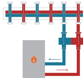
Горизонтальный монтаж гидравлического разделителя
