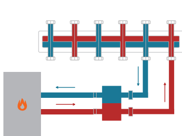
Вертикальный монтаж гидравлического разделителя
