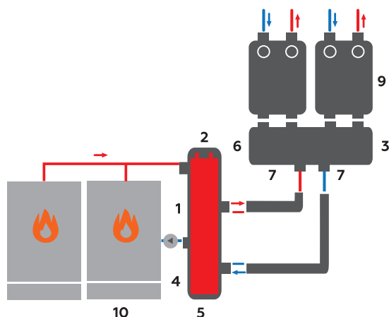
Вертикальный монтаж гидравлического разделителя
