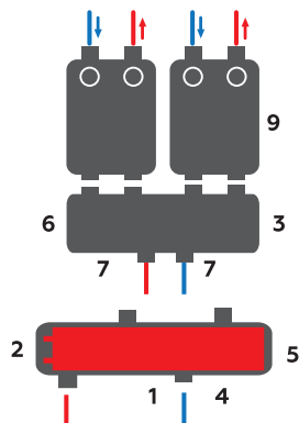
Горизонтальный монтаж гидравлического разделителя
